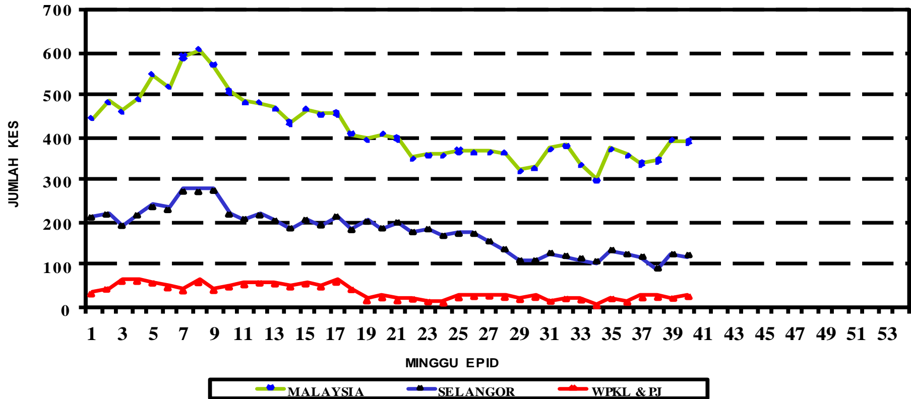
GRAF 2: MALAYSIA SELANGOR DAN WPKL & PJ KES MINGGUAN DENGGI 2012 (M.Epid 1 hingga 40)
