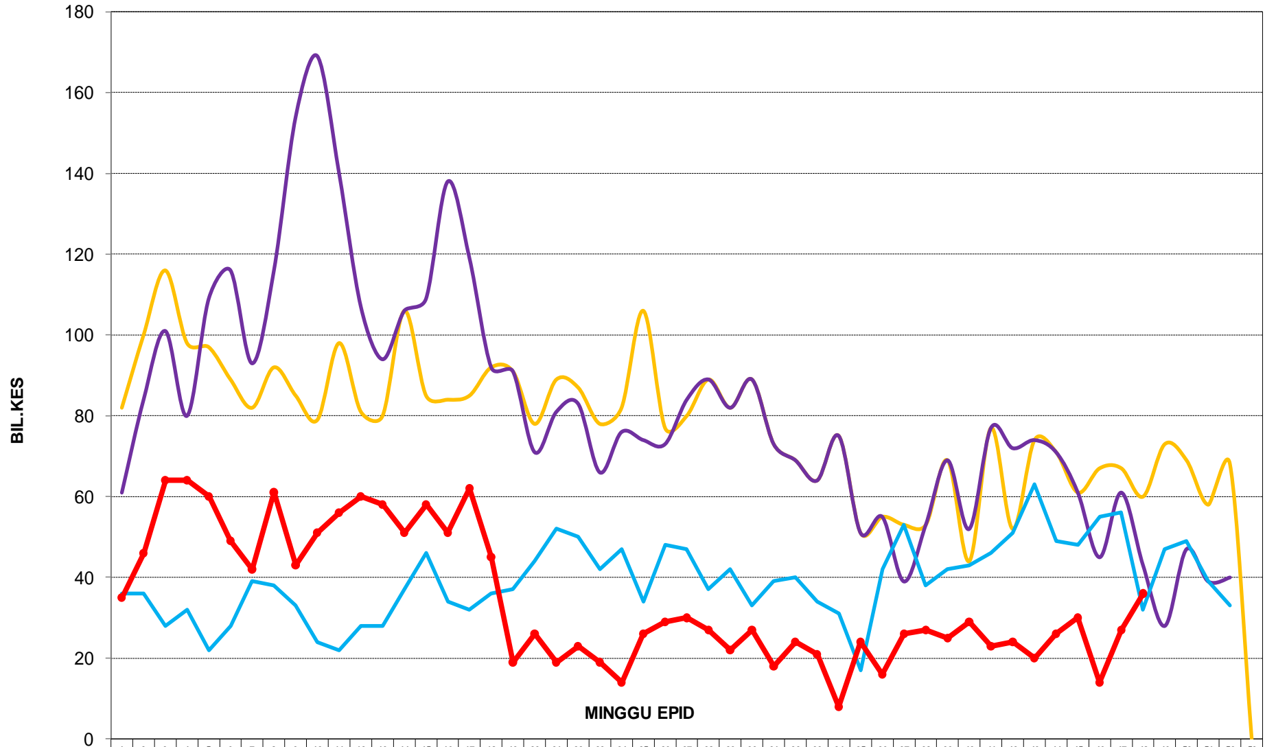
GRAF 1: TREND KES DENGGI MENGIKUT MINGGU EPID BAGI WILAYAH PERSEKUTUAN & PUTRAJAYA TAHUN 2010, 2011, 2012 DAN MEDIAN ( M.Epid 1 hingga 48)
